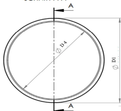
SCHNITT A-A
