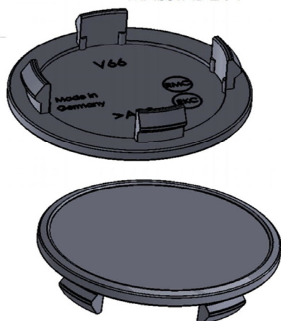
DETAIL B MABSTAB 2 : 1
