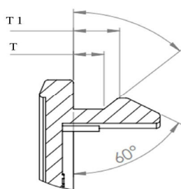
DETAIL B MABSTAB 2 : 1
